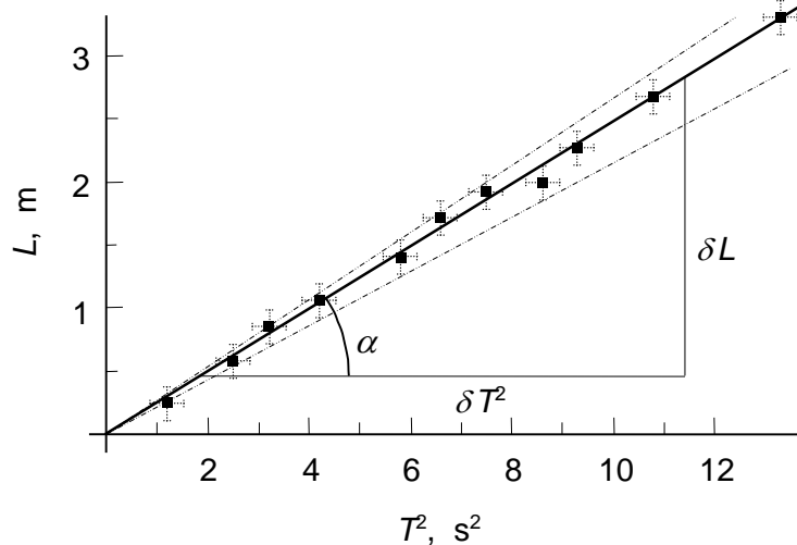
Fig. 2. Datos experimentales y ajuste visual de la ecuación (1).
