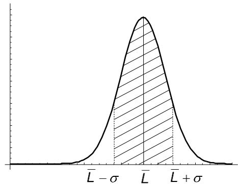
Fig. 1. Distribución normal de Gauss
